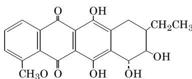
2 : Daunomycine
