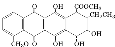
1 : Adriamycine
